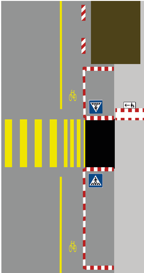
Provisorischer Fußgängerüberweg
